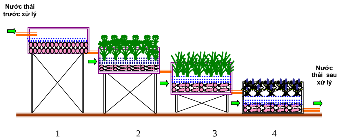
Hình 1. Sơ đồ quy trình xử lý nước thải ô nhiễm từ CBTBS
